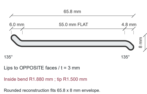
D Z SLAT PROFILE 1:1
