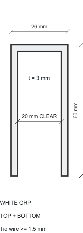
C U CAP 1:1
